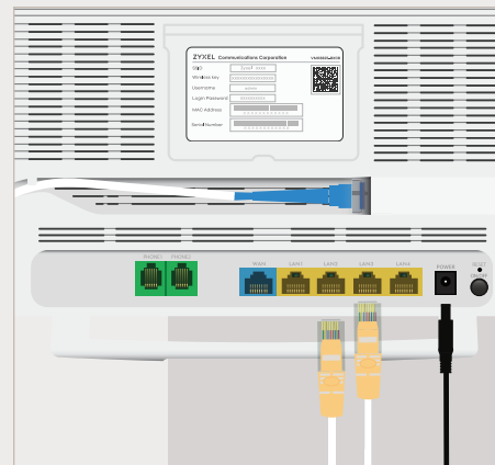
7. Flytt nettverkskablene fra den gamle hjemmesentralen, FMG, til de samme portene på den nye hjemmesentralen. Sett i strømmen og skru på hjemmesentralen.
